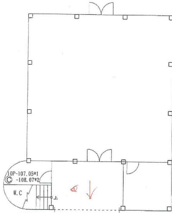
一樓平面圖
