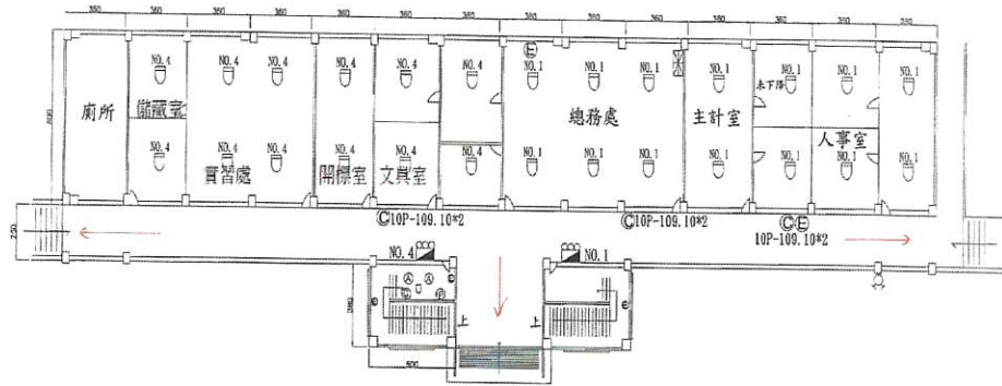
行政大樓 1F
