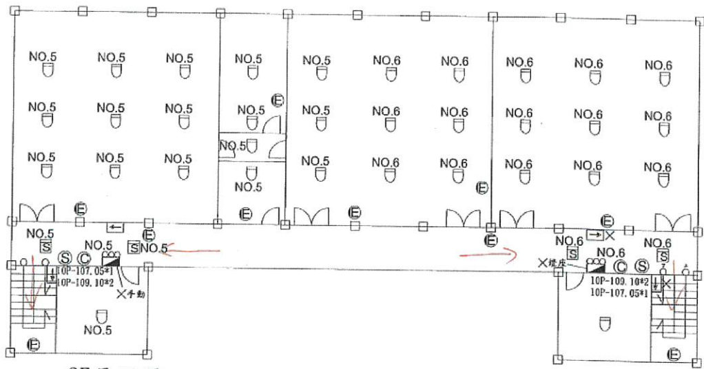
3F平面圖
