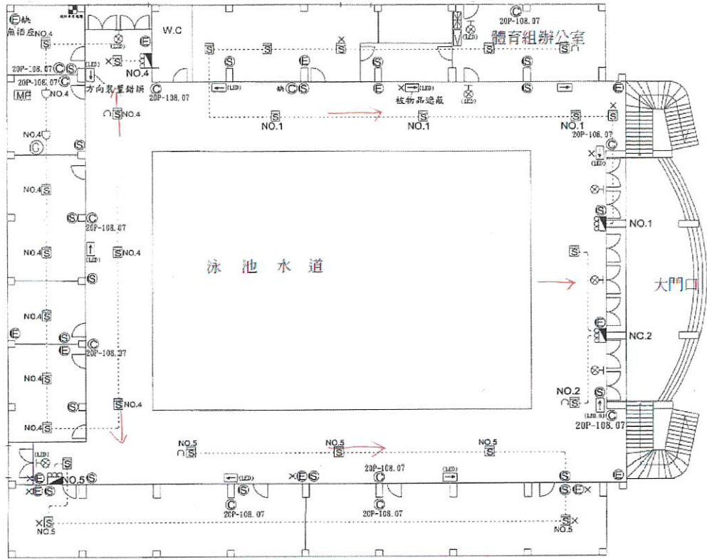
1F平面圖
