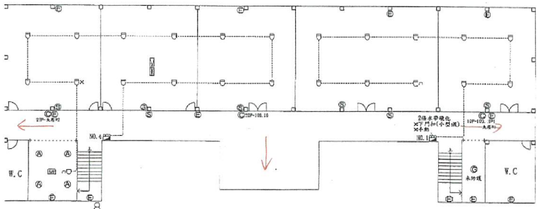
一樓平面圖
